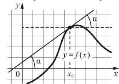
Геометрический смысл производной
